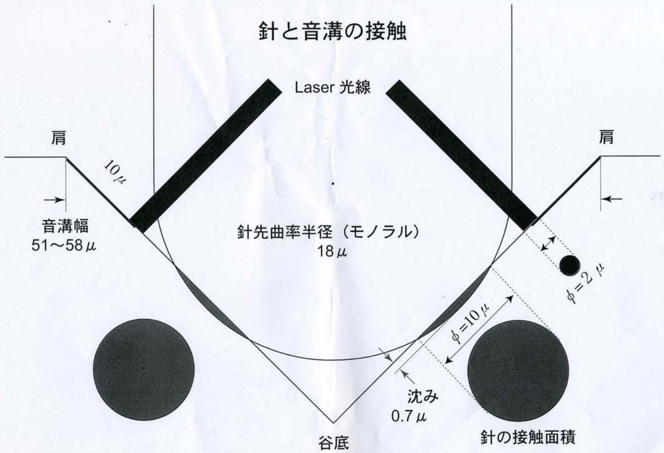
音溝断面図
