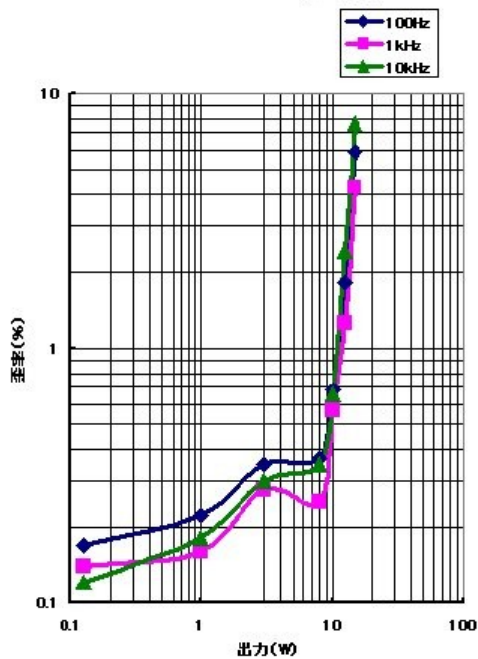
SATRIドライブ830Bシングルアンプ歪率 NF7dB
