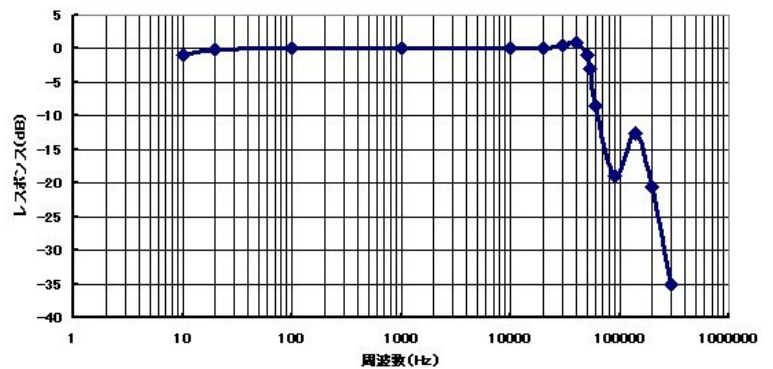
SATRI-DRIVE830Bシングルアンプ周波数特性(NF7dB)
